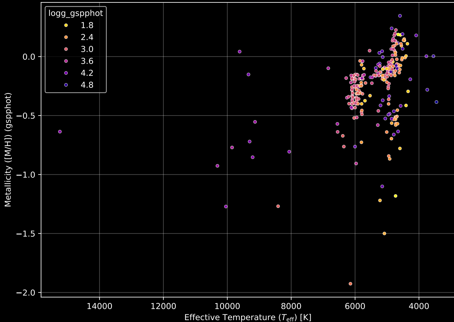
APOGEE DR17 Field: [N3201] Stellar Population Parameters (n= 249)
